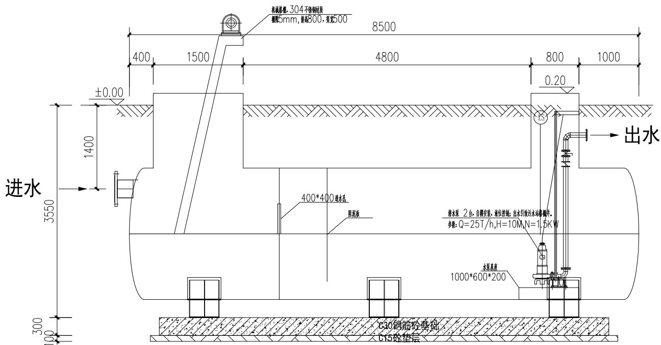
非标钢制一体化格栅提升井立面图
