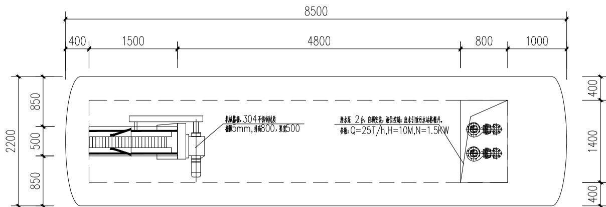
非标钢制一体化格栅提升井平面图
